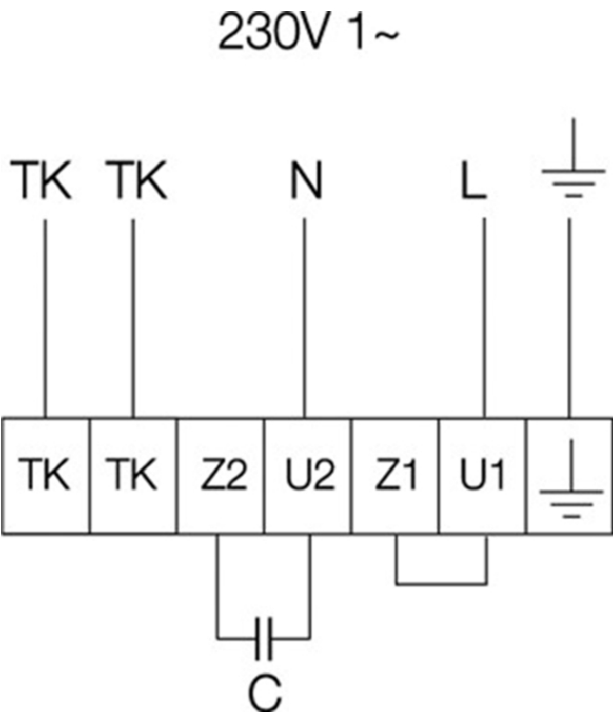
Схема подключения
